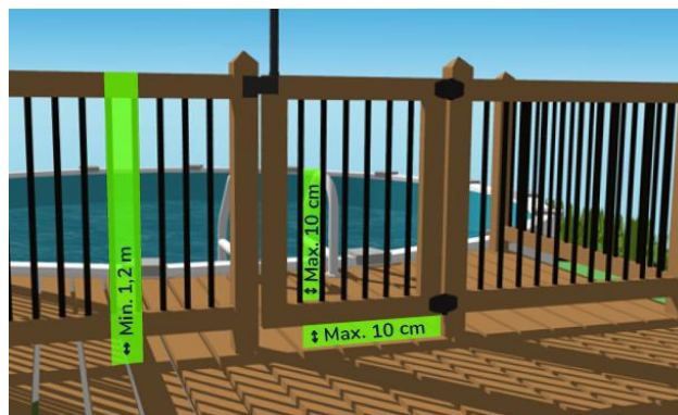
Figure 3 - Dimensions exigées pour une enceinte
